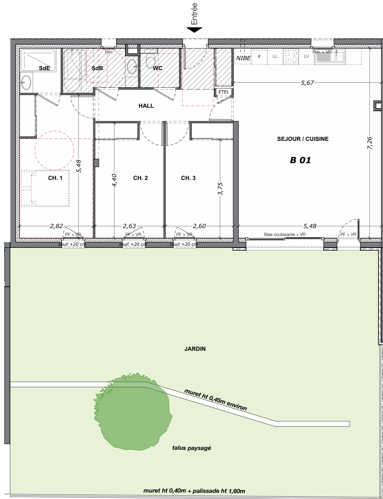
PLAN DU REZ DE CHAUSSEE
