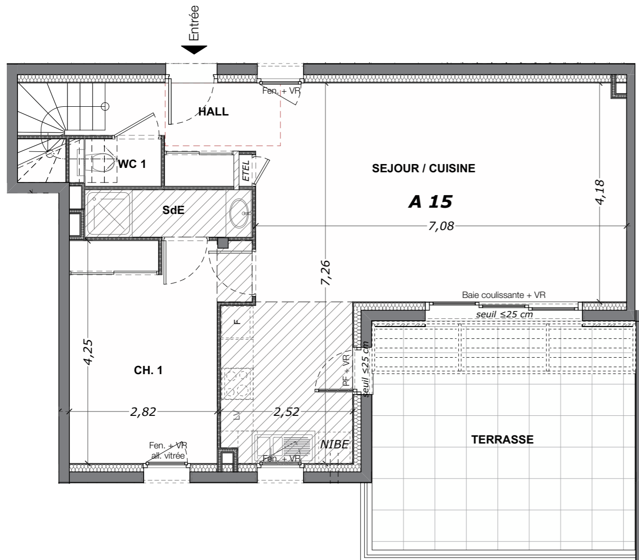
PLAN DU NIVEAU 1
